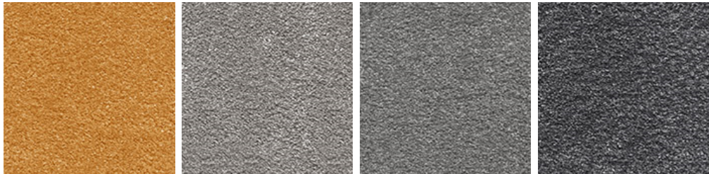
SIRIUS 54
